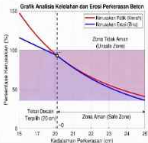
Gambar 2: Grafik Analisis Fatik dan Erosi Perkerasan Beton .
