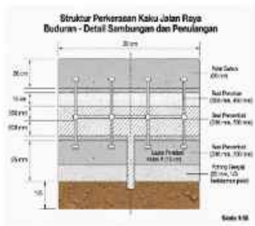
Gambar 3: Struktur Perkerasan Kaku Jalan Raya Buduran - detail sambungan dan penulangan.
